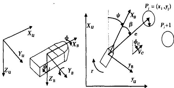
图 1 船舶动力自动定位原理示意图
