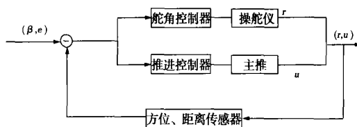
图 2 船舶动力控制系统结构图
